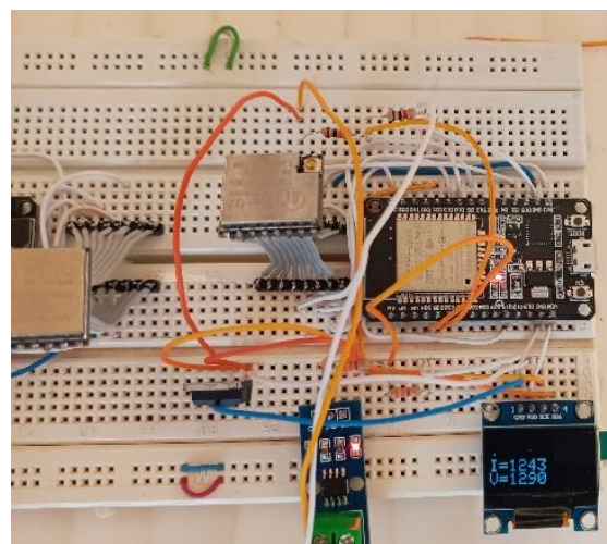
شکل (۳). سنسور جریان ACS712 متصل به میکروکنترلر و نمایش خروجی روی OLED به صورت خام
