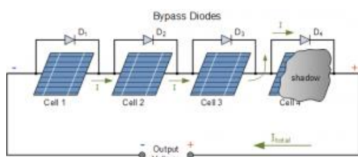
شکل (۱). نحوه‌ی اتصال پنل‌های خورشیدی به صورت سری به همراه دیودهای بای‌پس
