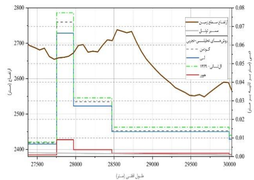
شکل (۱۲): مقایسه روش‌های تحلیلی-تجربی در تخمین دبی هجوم آب در تونل شمالی
