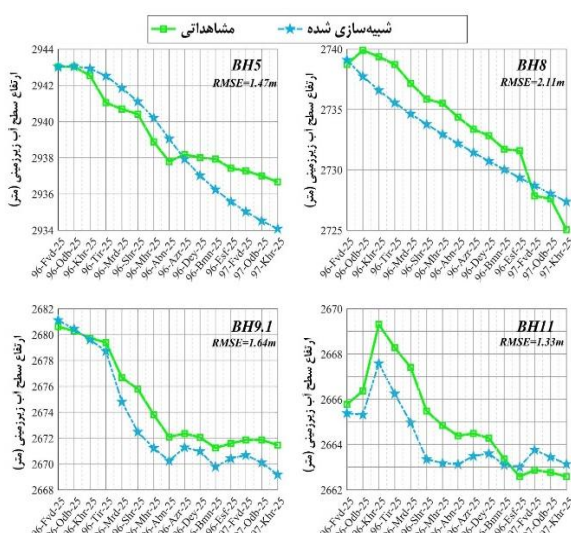
شکل (۷): نمایش ارتفاع سطح آب مشاهداتی و شبیه‌سازی شده
