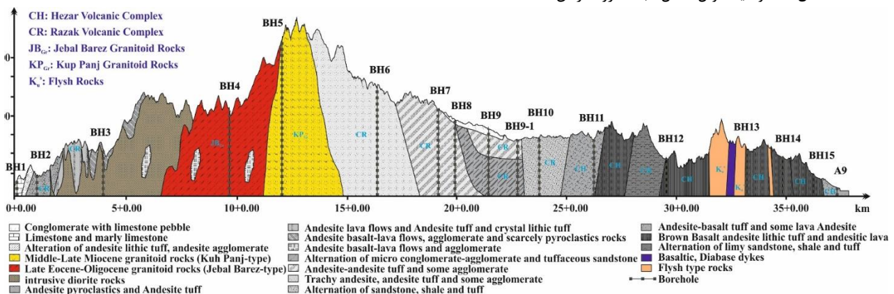
شکل (۳): مقطع عرضی زمین‌شناسی مسیر تونل
