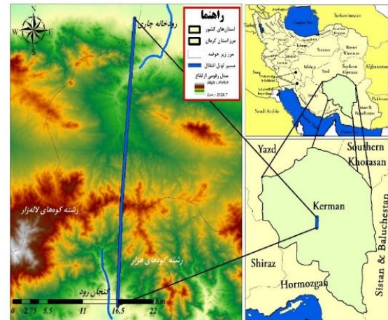
شکل (۱): موقعیت تونل انتقال آب صفارود کرمان
