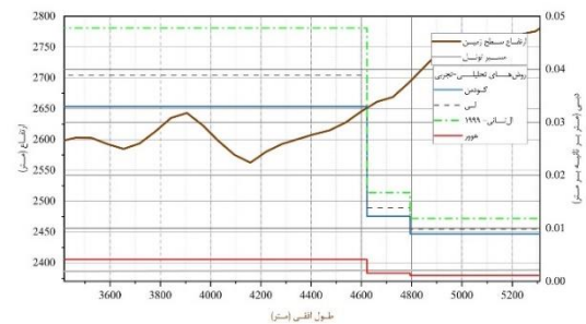
شکل (۱۳): مقایسه روش‌های تحلیلی-تجربی در تخمین دبی هجوم آب در تونل جنوبی
