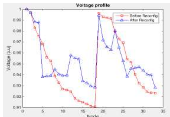
شکل (۶). پروفیل ولتاژ پس از بهینه‌سازی چندهدفه
