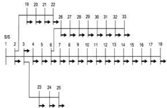
شکل (۱). شبکه ۳۳ باسه استاندارد IEEE
