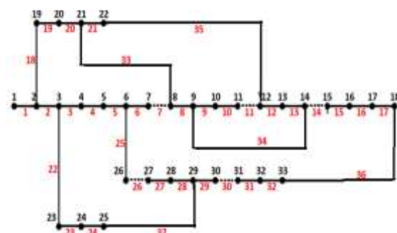
شکل (۸). ساختار شبکه پس از بازآرایی با الگوریتم MOPSO
