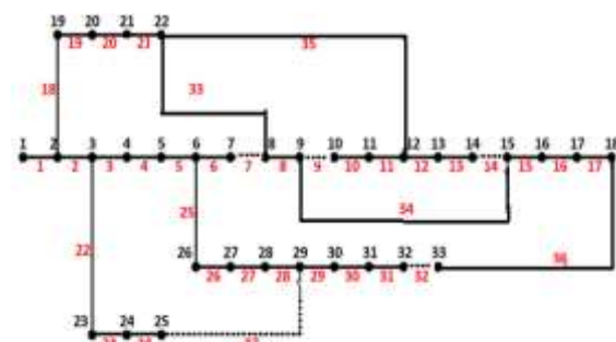
شکل (۷). ساختار شبکه پس از بازآرایی با روش تک هدفه
